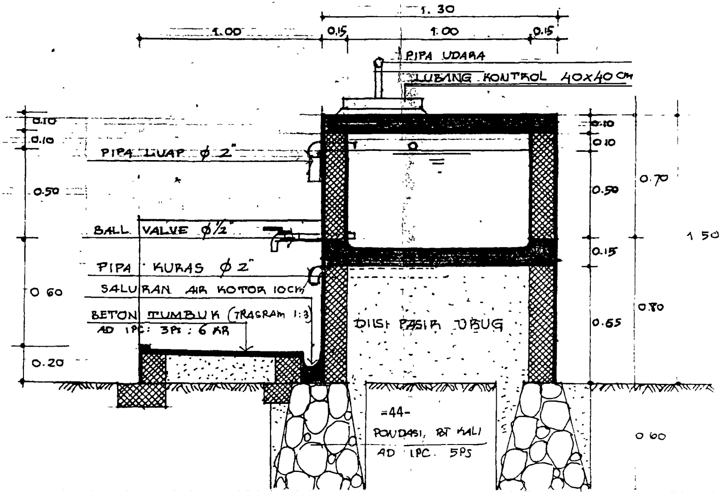
POT A-A SKALA 1:20
