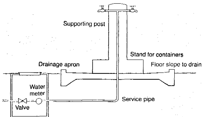
Fig. 3 Standpost.
