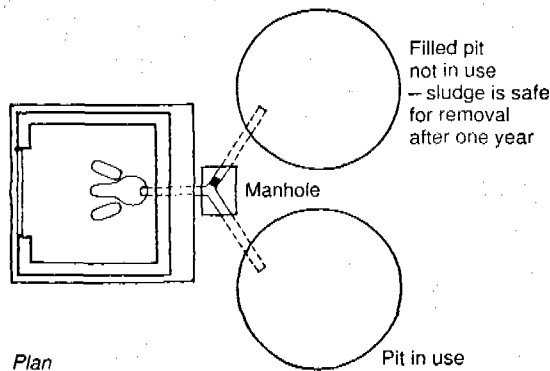
Fig. 4 A pour flush double pit latrine.
